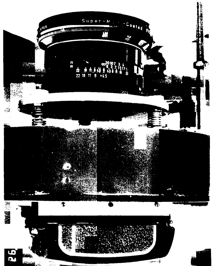
Het f/4.5-35 mm Pentax objektief is in drie punten instelbaar bevestigd. De sektor bevindt zich in de ronde trommel. Eronder de gemotoriseerde Mamiya achterwand.
