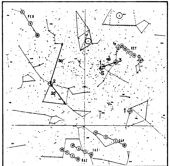
Figure 1: Wat een waarnemer moet weten: Standaard sterren, standaard afstanden ( 10^\circ 30^\circ ), de posities van de radianten van de zomerzwermen en de belangrijkste grensmagnitude-gebieden.
