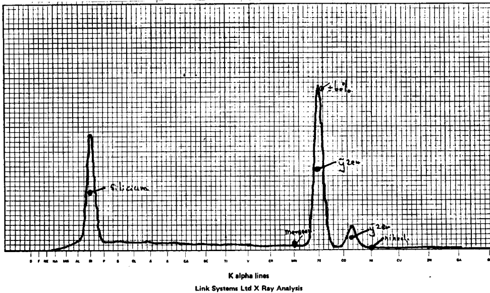
Figure 4: Röntgen spectrum van een geanalyseerd gebiedje van 50x50 µm, met resonantielijnen van silicium, ijzer en sporen van mangaan en nikkel (T.U.Twente, W.H.J.Bruis).
